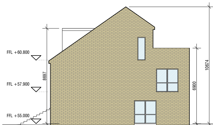
RHS ELEVATION - TYPE E1 SCALE 1:200
